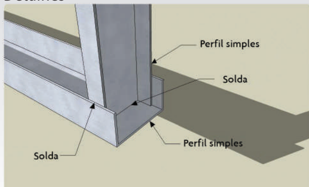
Solda de perfis simples
