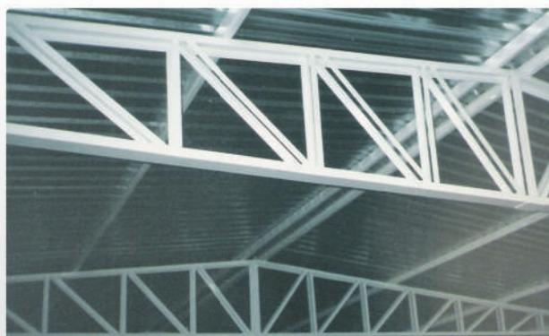
Perfil simples e cantoneira
