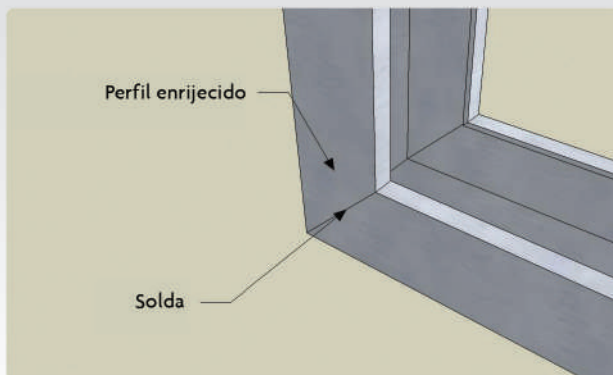
Solda de perfis enrijecidos
