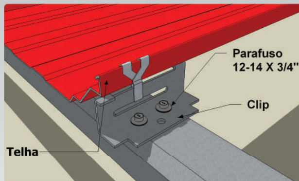
Colocação da primeira telha zipada
