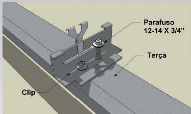
Clip de fixação de telha zipada
