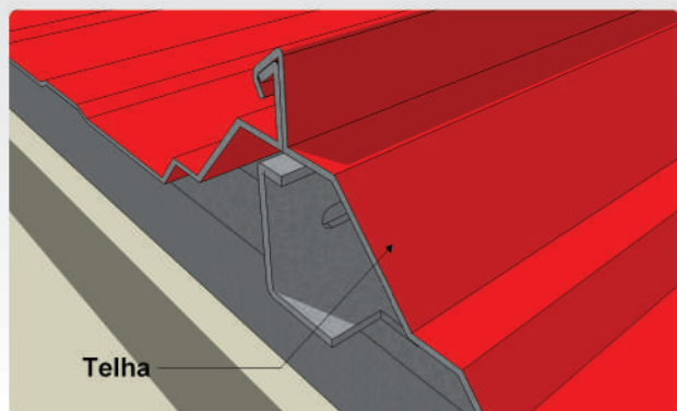
Colocação da segunda telha zipada
